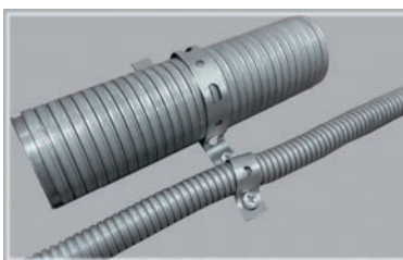
Приклад кріплення металорукава різних Ду за допомогою перфострічки
