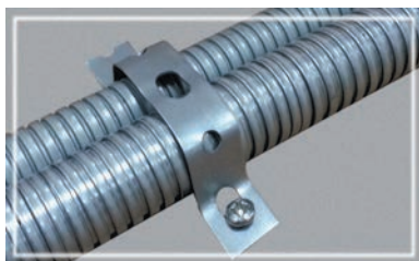
Приклад кріплення металорукава двох і більше Ду за допомогою перфострічки
