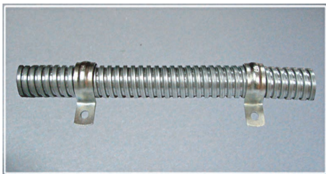
Приклад кріплення металорукава за допомогою скоби монтажної металевої
